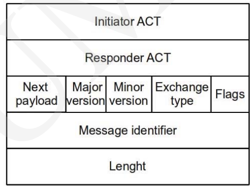
Fig. 2. ISAKMP header.
